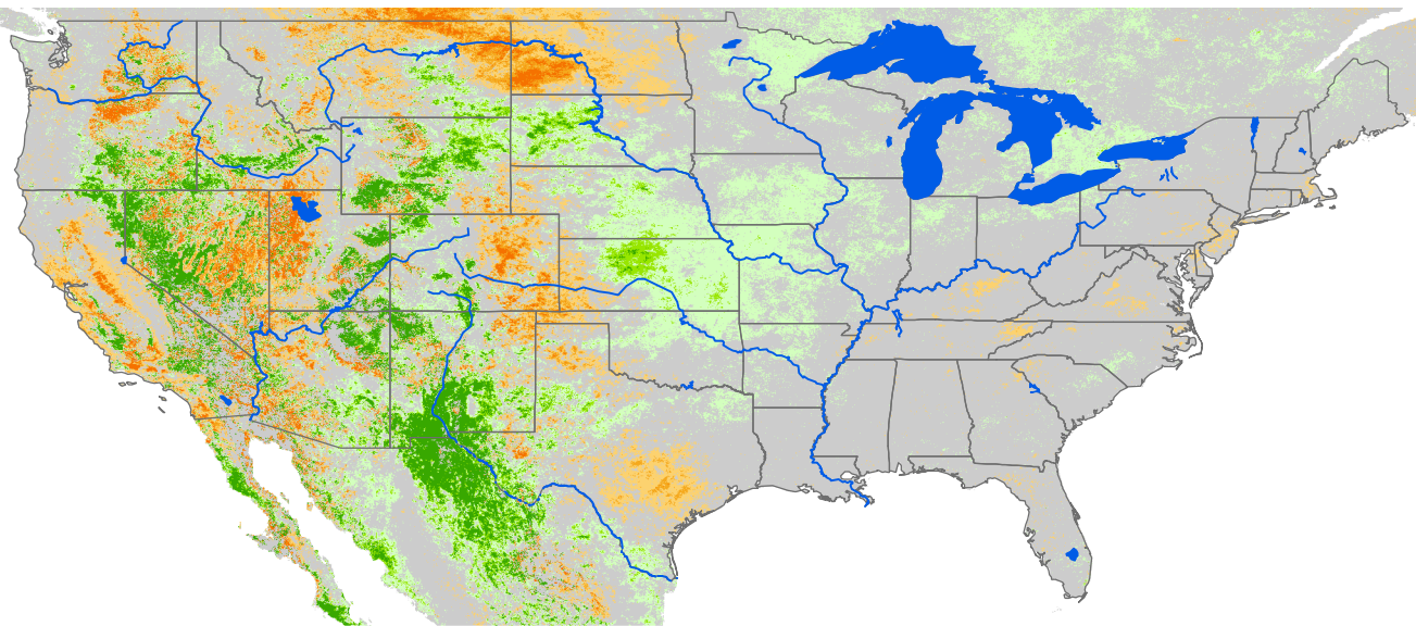
ET Anomaly (%)
